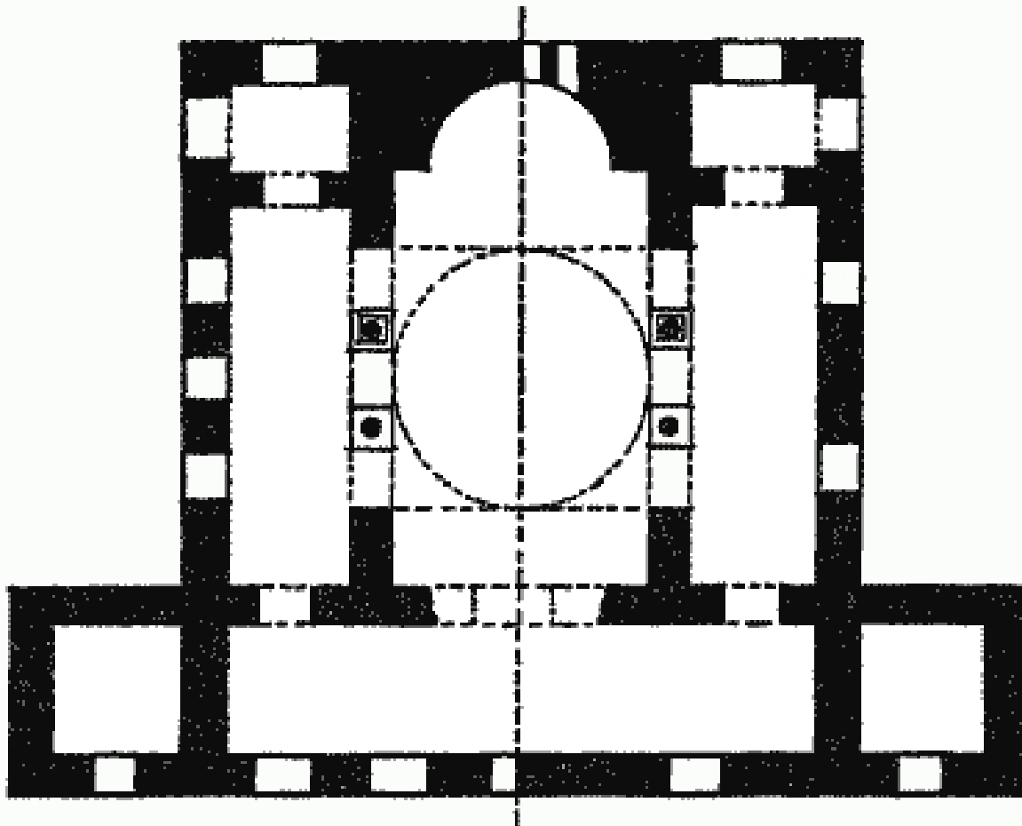
Fig. 1.—Kasr Ibn Wardan (Strzygowski).
