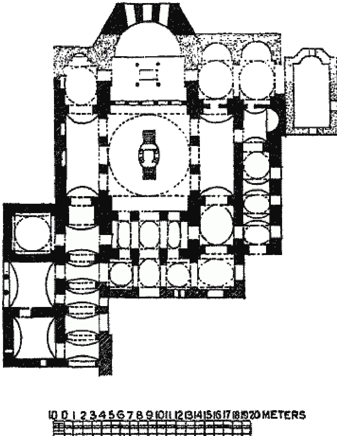
Fig. 4.—S. Nicholas, Myra (Rott).
