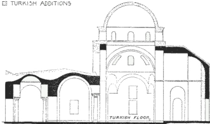
LONGITUDINAL SECTION
